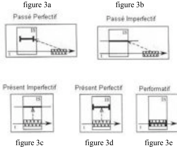
Figure 3. — (Langacker 1995 : 225)
