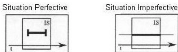
Figure 2. — (Langacker 1995 : 224 2 )
